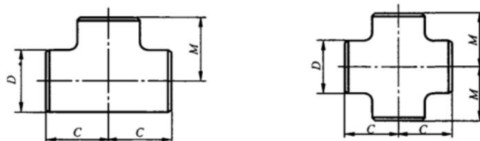
图 7 等径三通和四通
