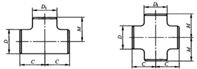
图 8 異径三通和四通
