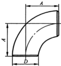
图 4 短半径 90°弯头
