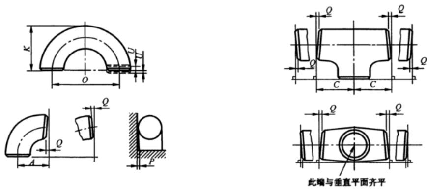
图 14 公差简图
