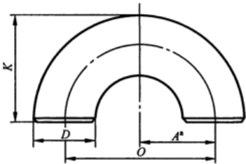
图 5 短半径 180°弯头
