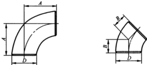
图 1 长半径 90°和 45°弯头
