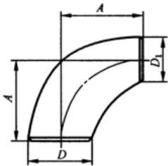
图 2 90°长半径异径弯头
