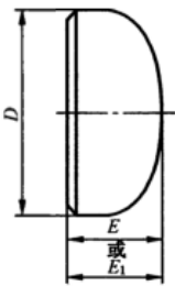
图 10 管帽
