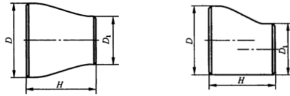
图 11 异径管
