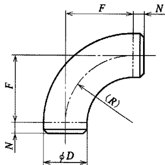
ネック付き 90° エルボ (両ネック)
