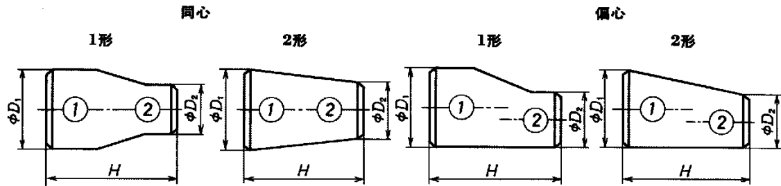
付表 4 レジューサの形状・寸法
