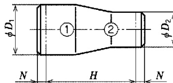
同心1形
