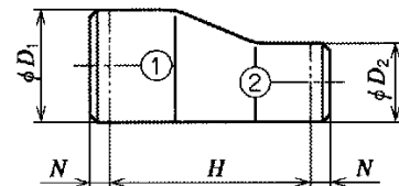
偏心1形
