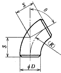
附属書付図1 特殊角度エルボ
