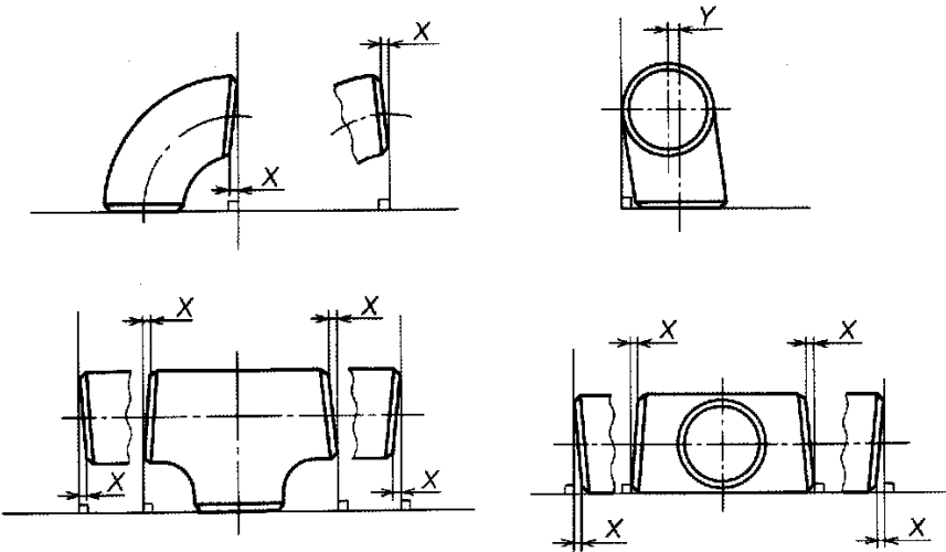
付表 8 管継手の直角度の許容値
