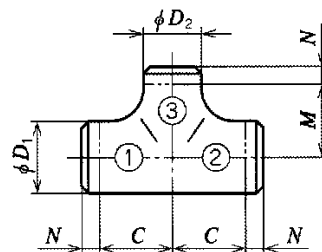
径違い
