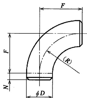
ネック付き 90° エルボ (片ネック)
