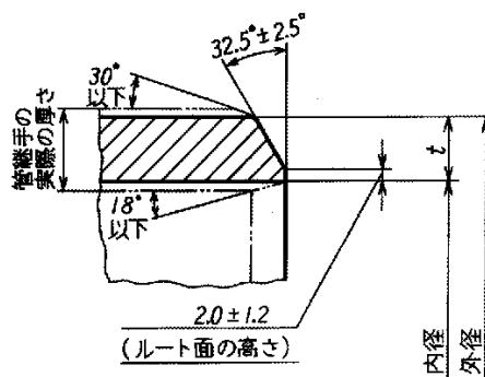
図 1 ベベルエンドの形状・寸法
