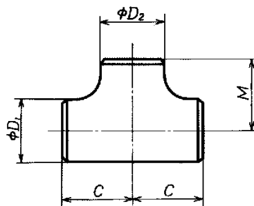
付表 5 同径 T の形状・寸法
