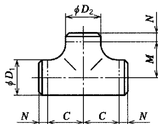
同径
