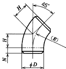
ネック付き 45° エルボ (片ネック)
