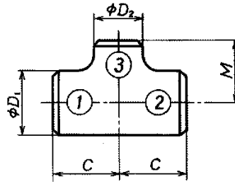
付表 6 径違い T の形状・寸法
