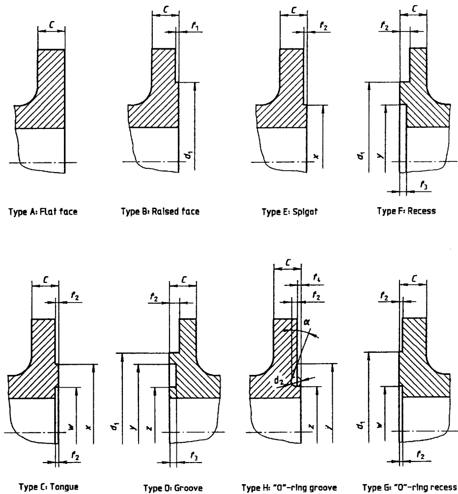
Figure 6 — PN 2,5, PN 6, PN 10, PN 16, PN 25 and PN 40 flange facing dimensions
