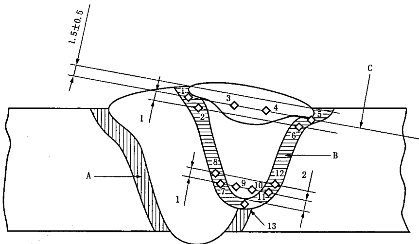
图 3 角焊缝
